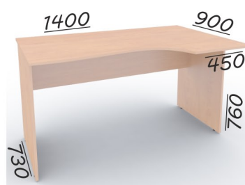
Стол эргономичный А-200 ПРАВЫЙ
